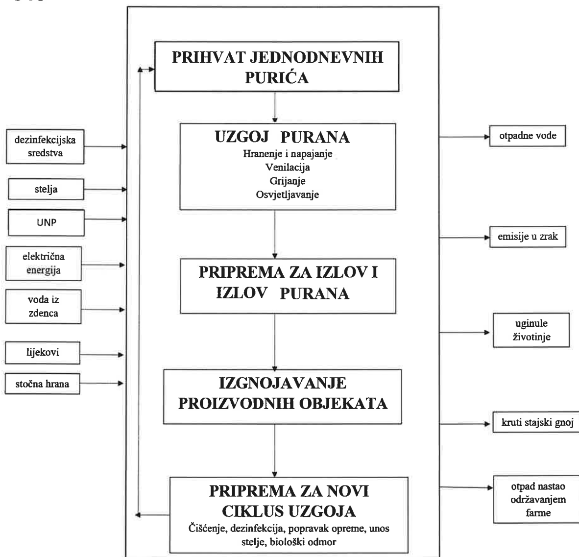
Prilog 2. Bok dijagram tehnološkog procesa na postojećem postrojenju za intenzivan uzgoj peradi Farma 11
